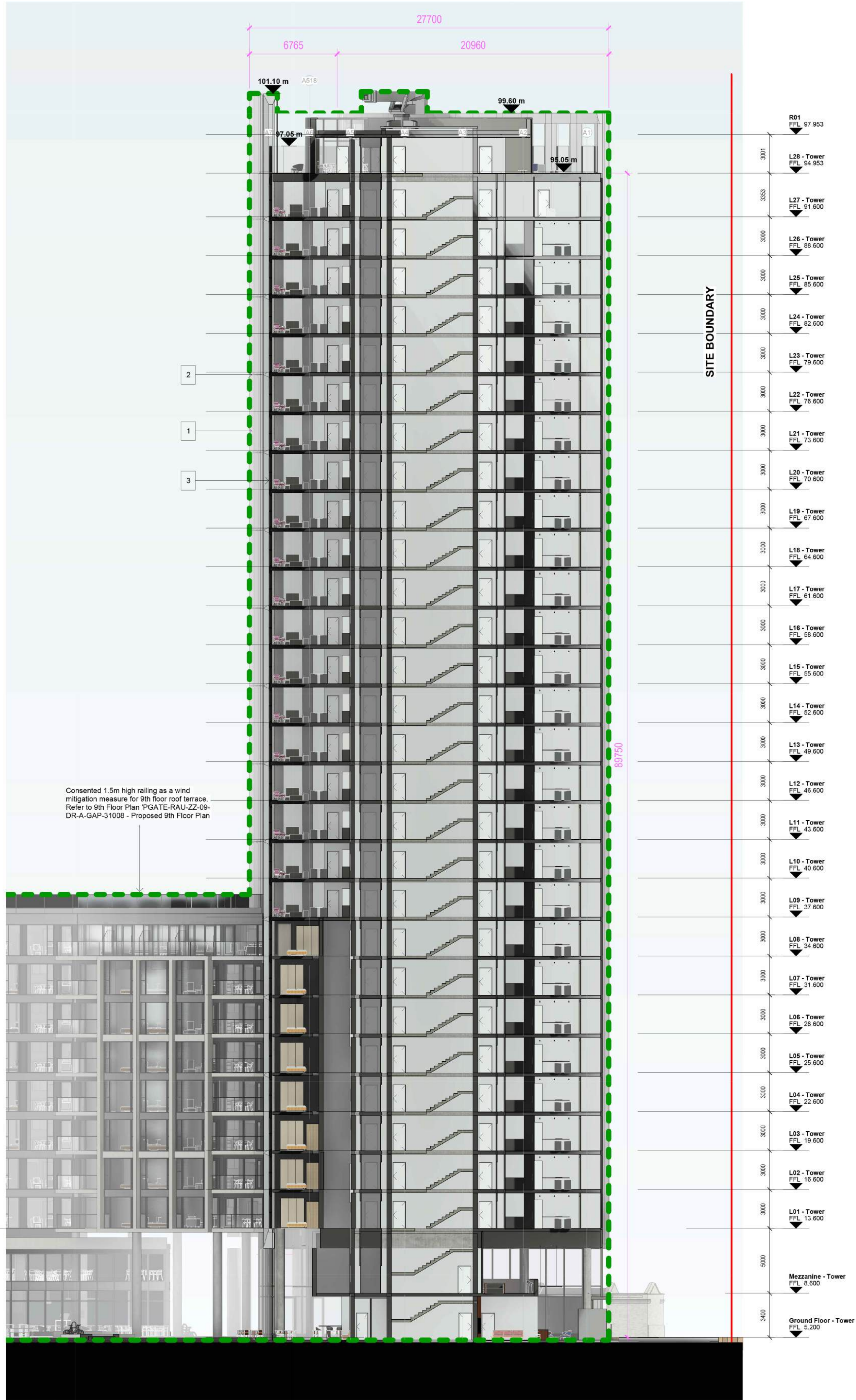
Section CC 1 : 200
