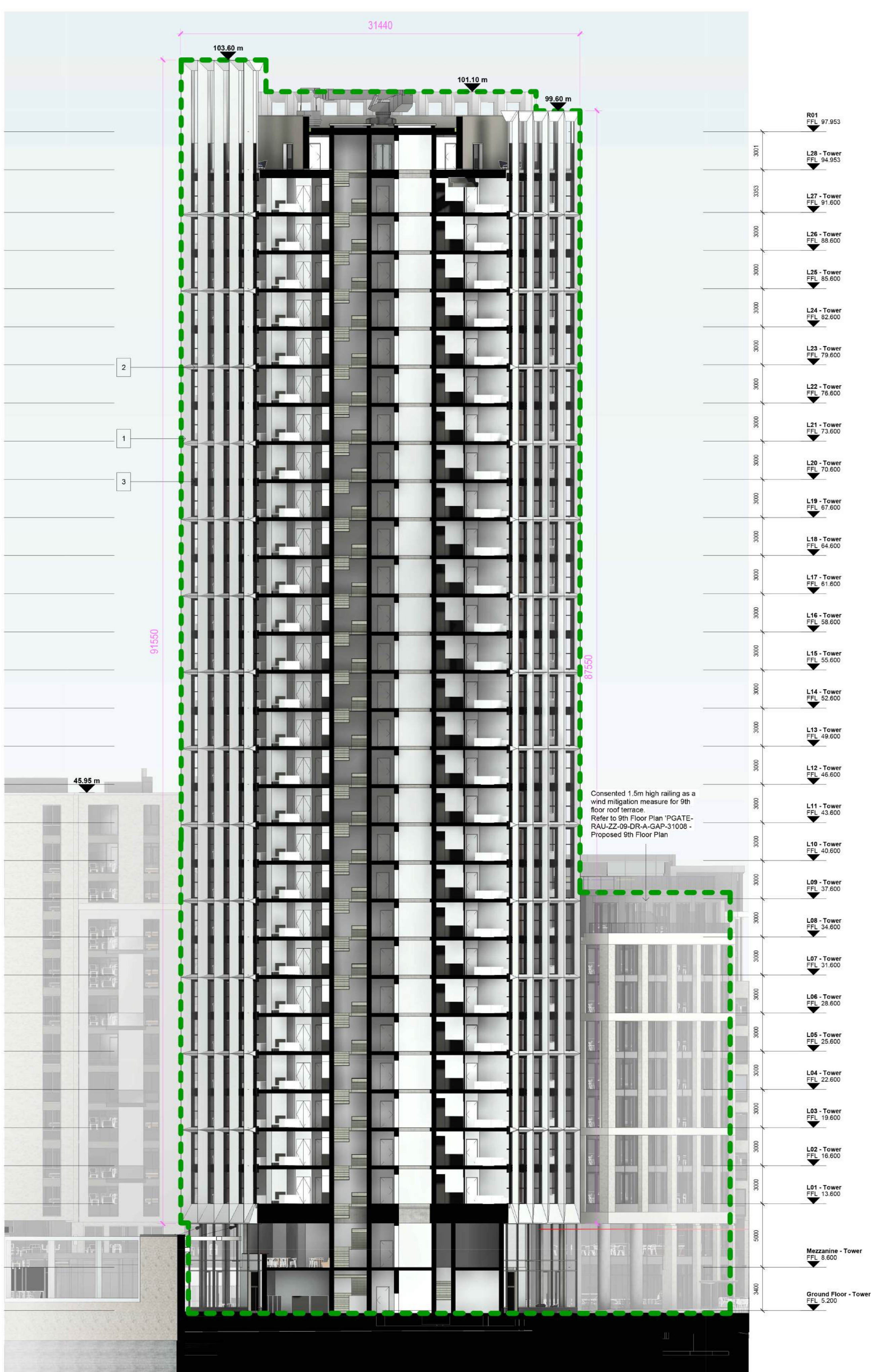
Section DD 1 : 200
